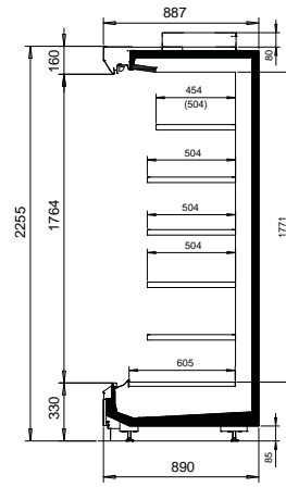
TectoDeck MD5 30-89-226
