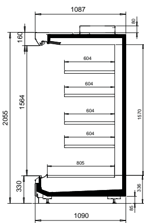
TectoDeck MD5 30-109-206
