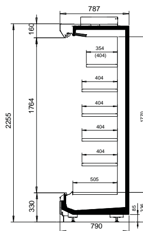
TectoDeck MD5 30-79-226
