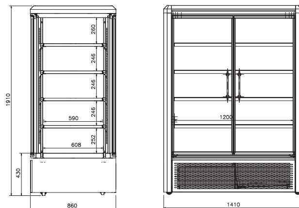
Zweiseitiges steckerfertiges Kühlregal TectoPromo MD4 Visio
