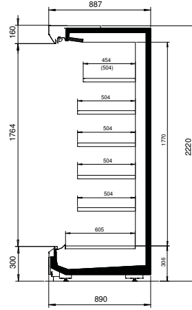
TectoDeck MD5 30-89-222
