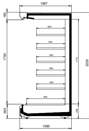
TectoDeck MD5 30-109-222
