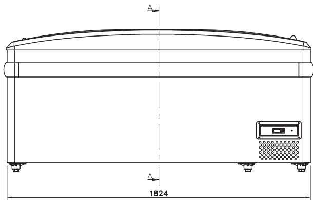
TectoFreeze IS2 183-FC-CE °C от -23 до -18 °C / -от -1 до +5 °C
