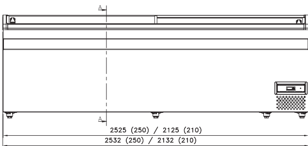
TectoFreeze IS2 210-F °C от -23 до -18 °C
