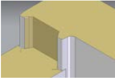
TectoCell Standard Plus -mallin raoton limitys helpottaa puhdistusta ja parantaa hygieniaa.
