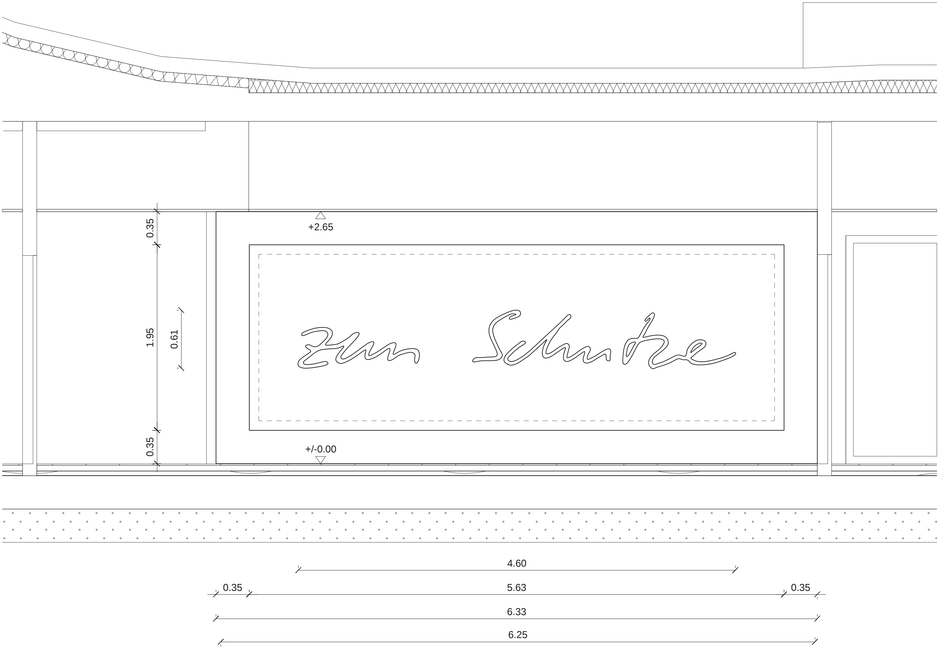
schnitt 3-3
