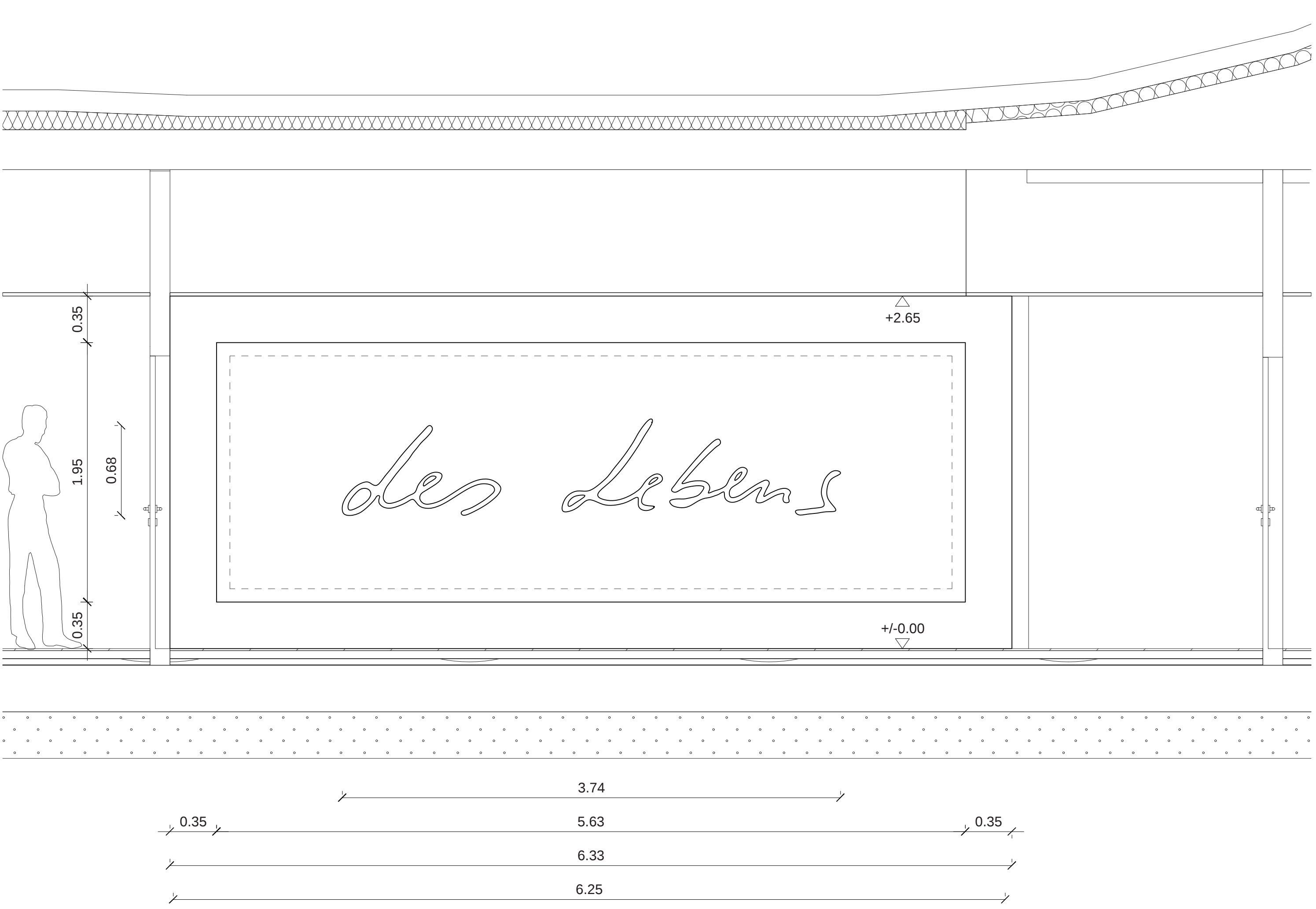
schnitt 2-2
