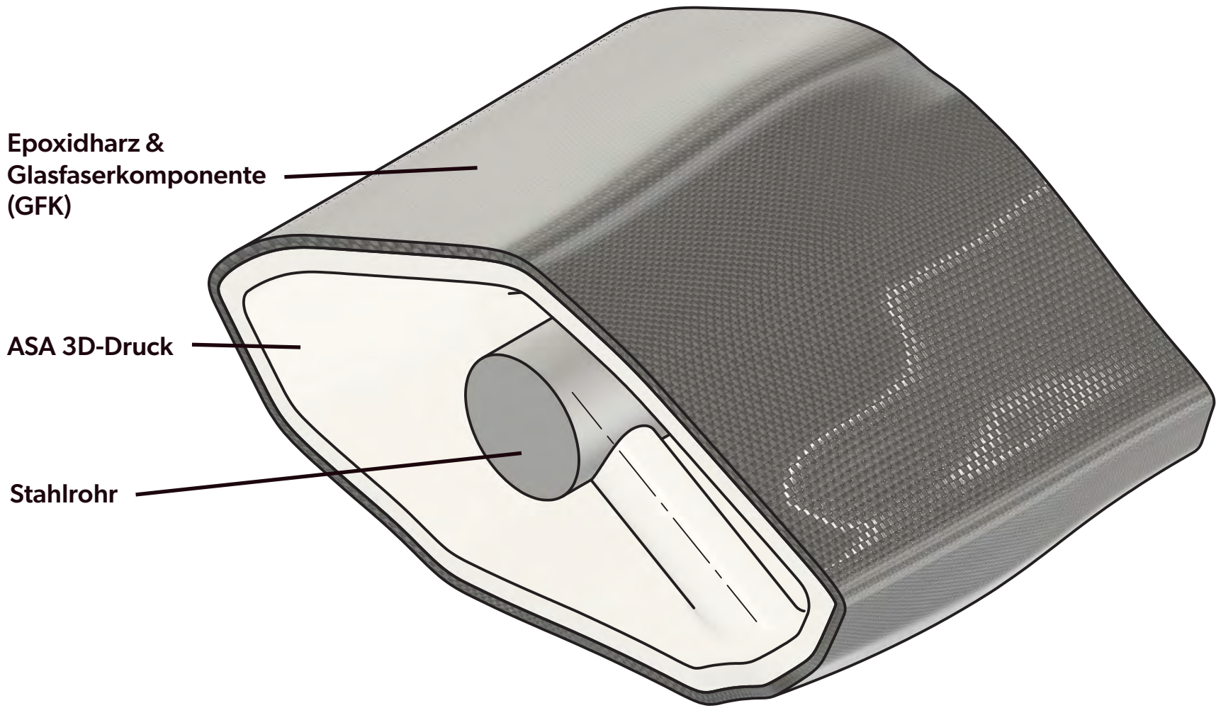
Querschnitt Rotorflügel
