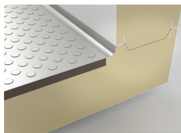
Congés de sol entièrement hygiéniques
