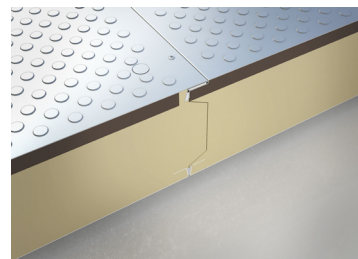
Assemblage des panneaux de sol avec recouvrement
