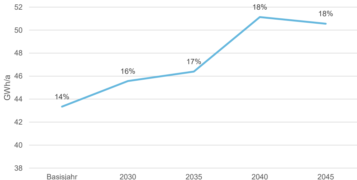
Abbildung 49: Anteil der Wärmenetze am Gesamtwärmebedarf im Zielszenario
