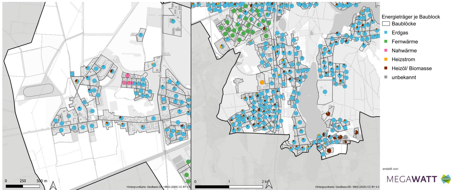
Abbildung 58: Dezentrale eingesetzte Energieträger je Baublock in Diepensee (links) und Zeesen (rechts)
