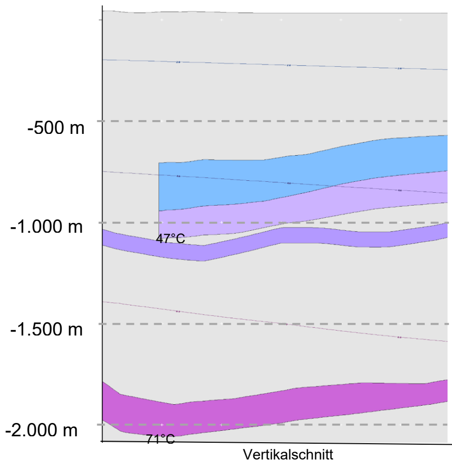
Abbildung 30: Erwartete Temperaturniveaus in Königs Wusterhausen 18
