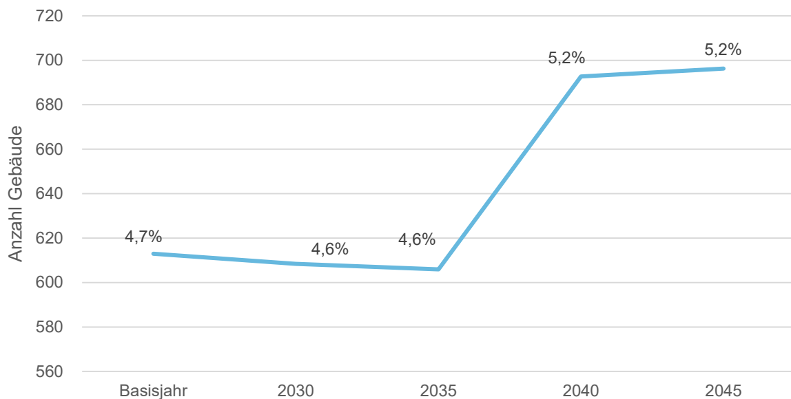
Abbildung 50: Anzahl der Gebäude am Wärmenetz und Anteil am gesamten Gebäudebestand
