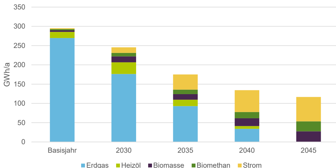
Abbildung 46: Entwicklung der Endenergieverbräuche im Zielszenario nach Energieträgern
