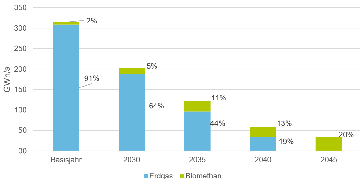
Abbildung 51: Entwicklung des Endenergieverbrauchs aus Gasnetzen im Zielszenario [MWh/a]
