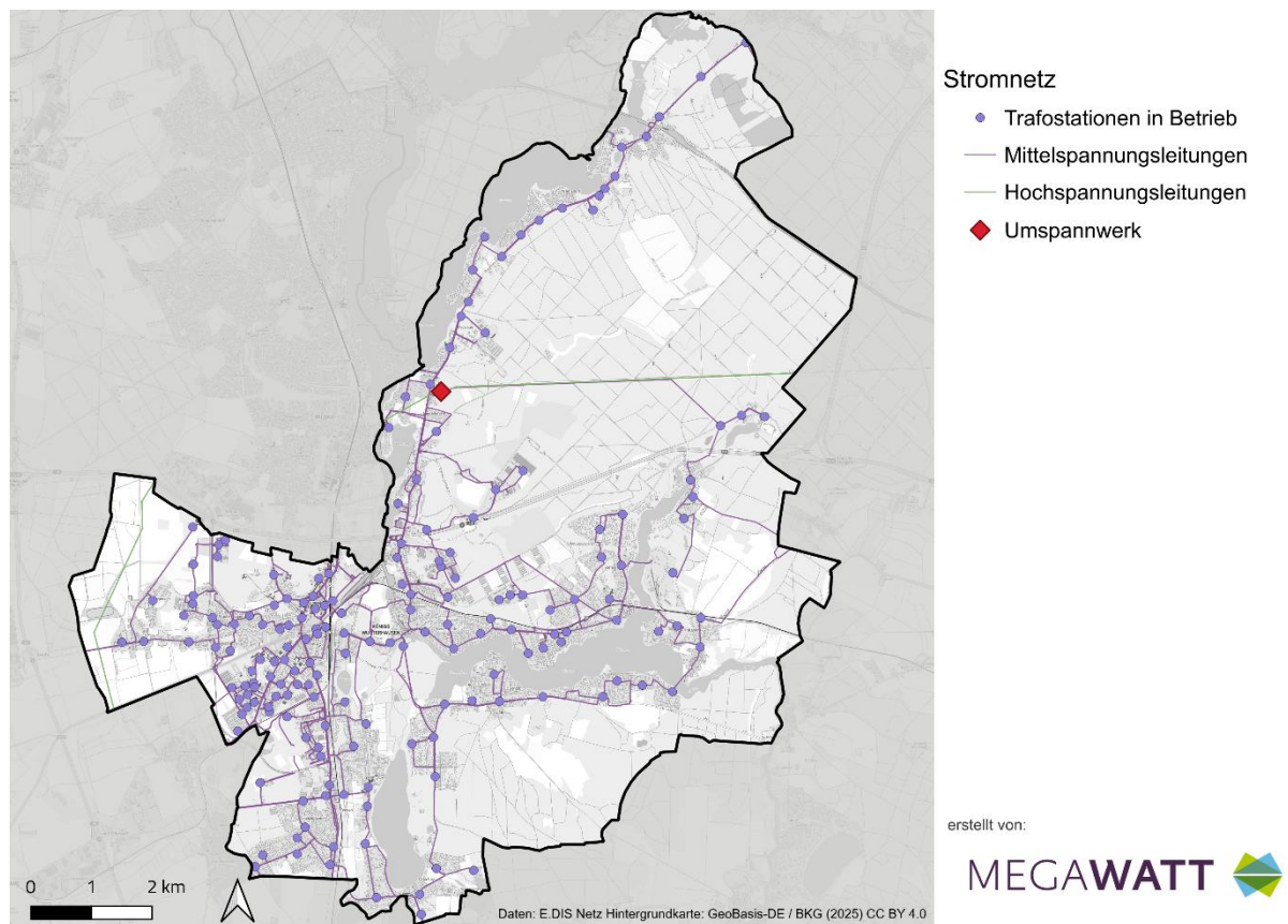
Abbildung 19: Strominfrastruktur in Königs Wusterhausen
