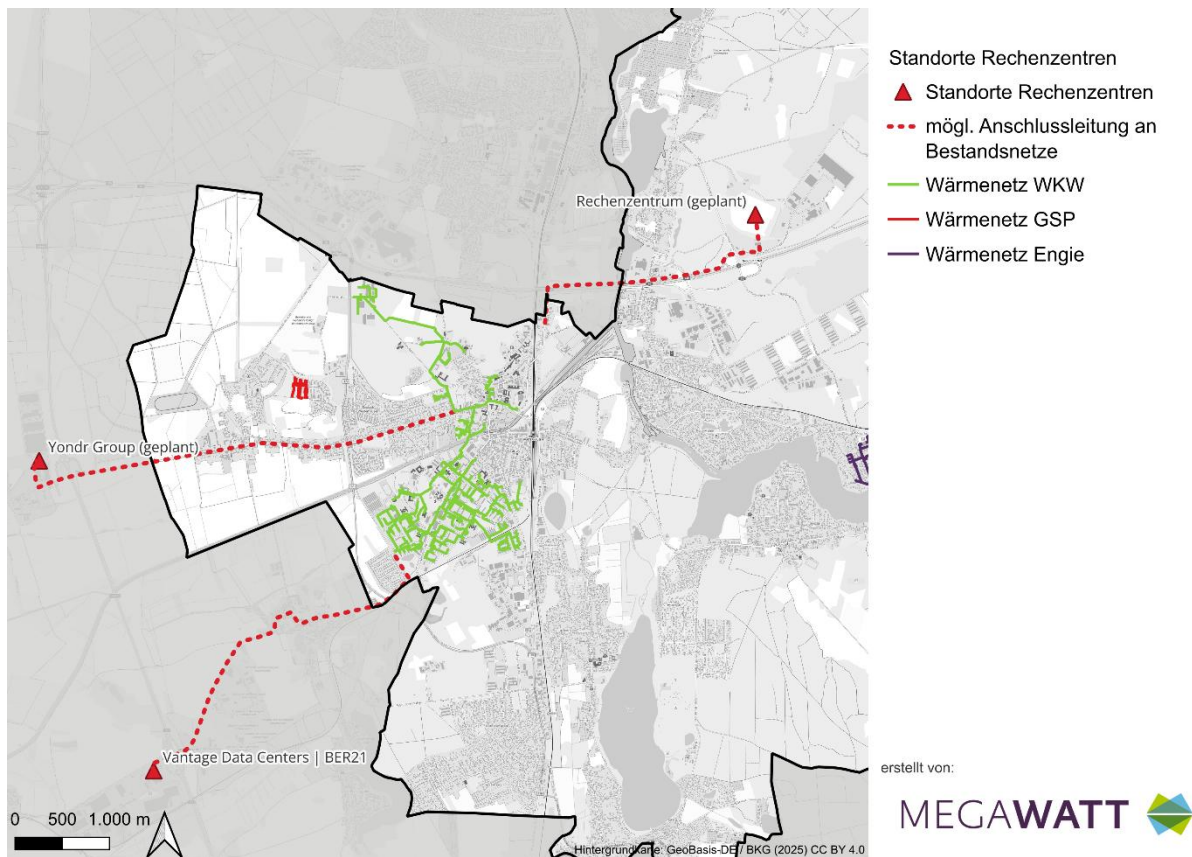
Abbildung 32: Standorte und mögliche Erschließung des Abwärmepotenzials der bestehenden und geplanten Rechenzentren
