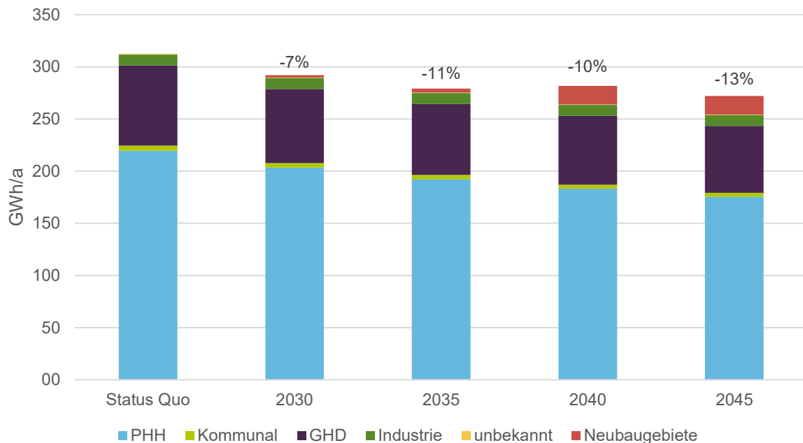
Abbildung 20: Entwicklung Wärmebedarf nach Sektoren [GWh/a]
