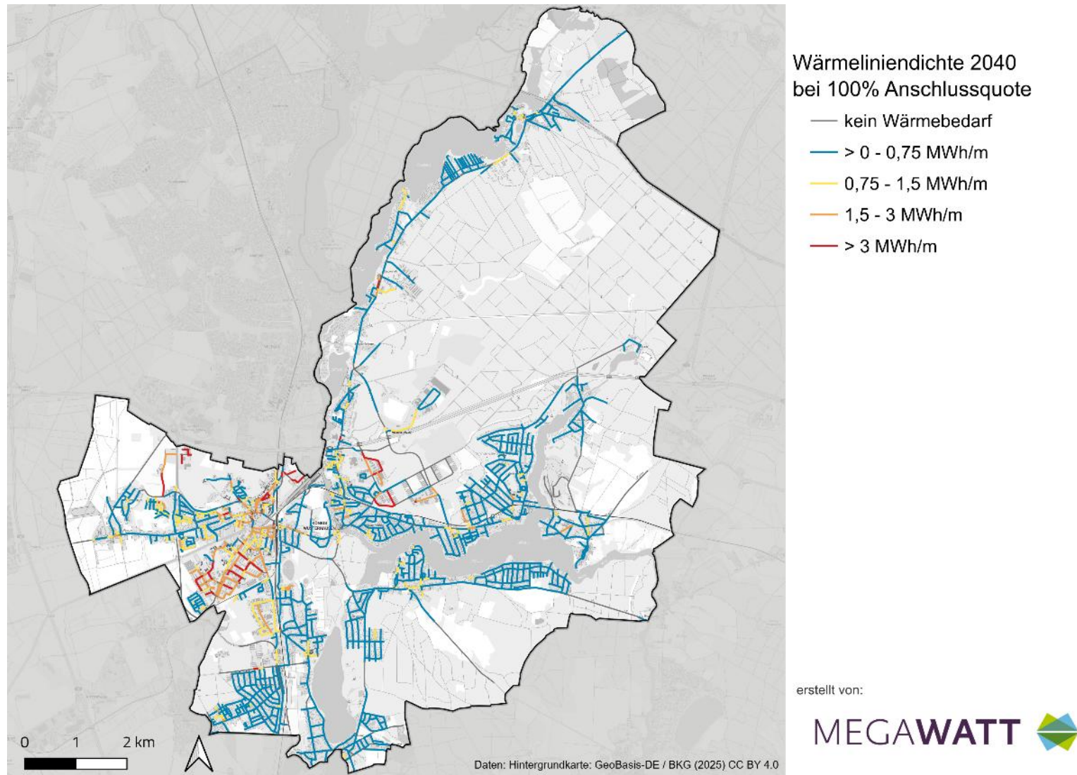
Abbildung 61: Wärmeliniendichte 2040 mit Anschlussquote 100%
