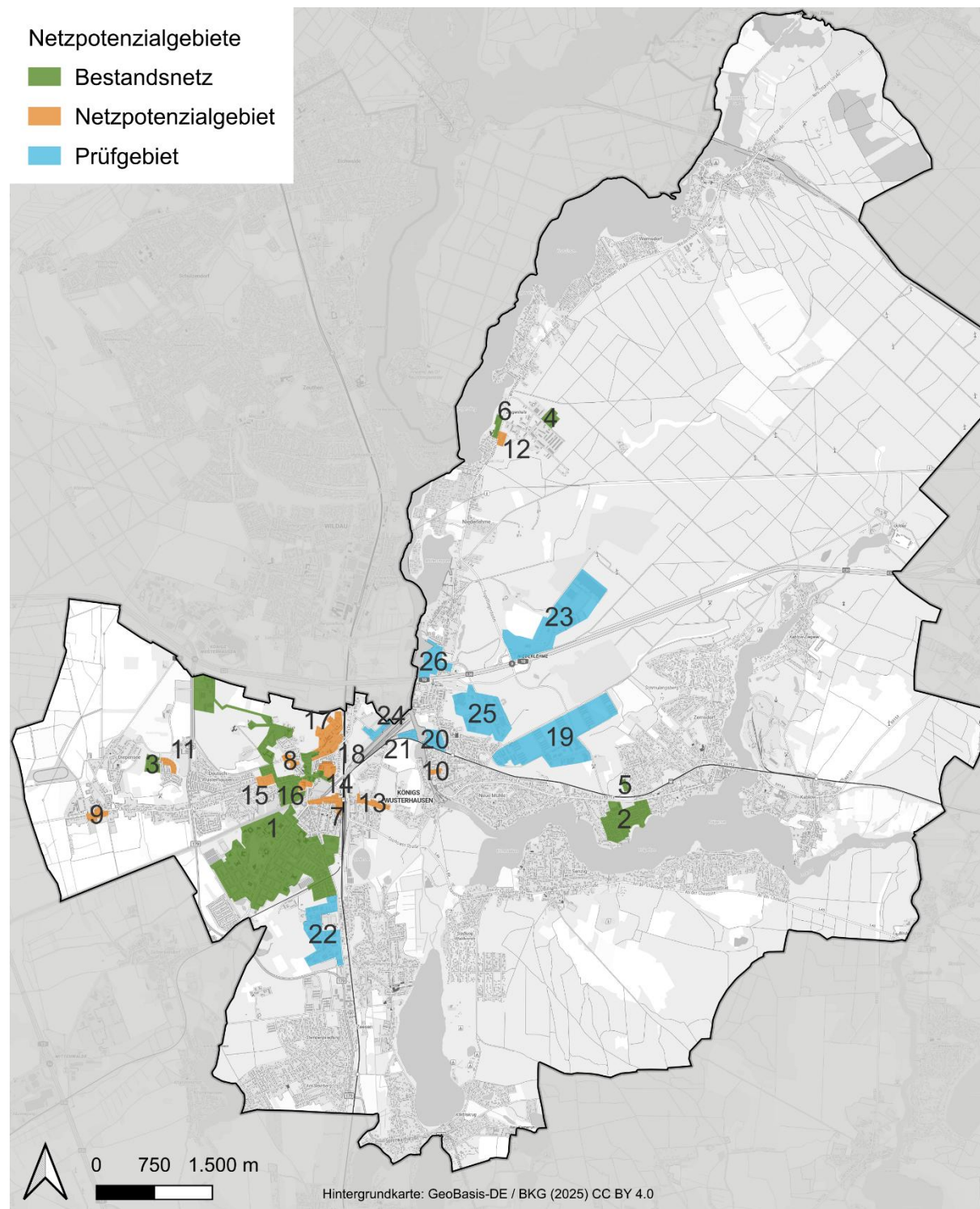
Abbildung 39: Netzpotenzialgebiete Königs Wusterhausen
