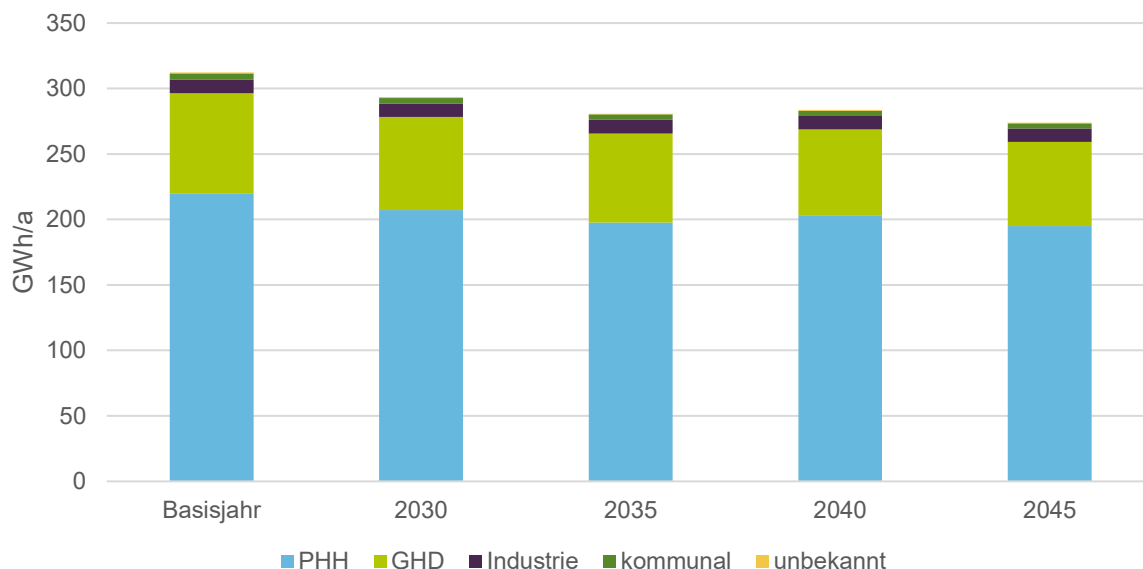
Abbildung 45: Jährlicher Wärmebedarf nach Sektoren
