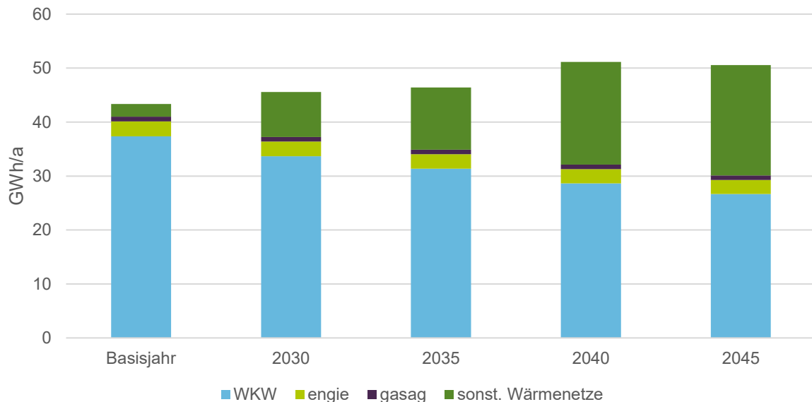
Abbildung 48: Entwicklung der Wärmebedarfe aus Wärmenetzen im Zielszenario
