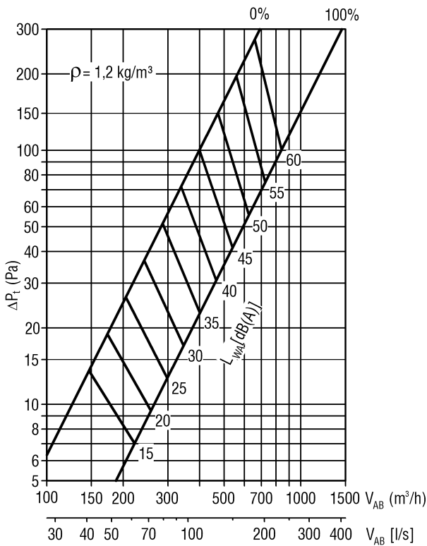
LWD-Q-A-6-...-00625-125-...-AK-80-...-S0
