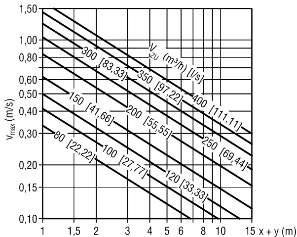
LWD-Q-Z-6-...-00625-225-...
