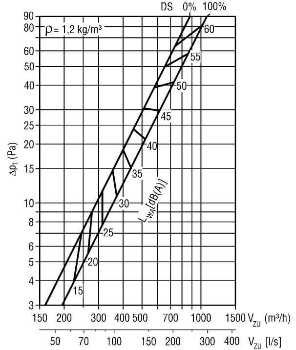
LWD-Q-Z-6-...-01025-225-...-AK-58-...-S1
