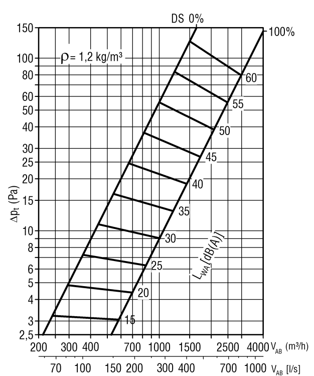
LWD-Q-A-6-...-01025-225-...-AK-80-...-S0
