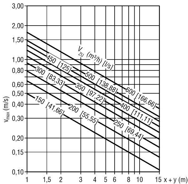
LWD-Q-Z-6-...-00625-225-...
