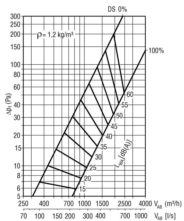
LWD-Q-A-6-...-01025-225-...-AK-80-...-S1
