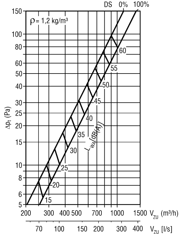
LWD-Q-Z-6-...-01025-225-...-AK-58-...-S0
