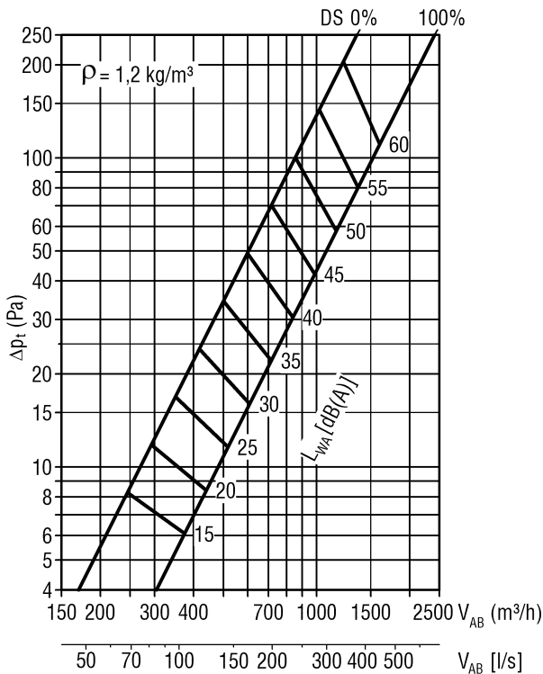
LWD-Q-A-6-...-01025-125-...-AK-80-...-S0
