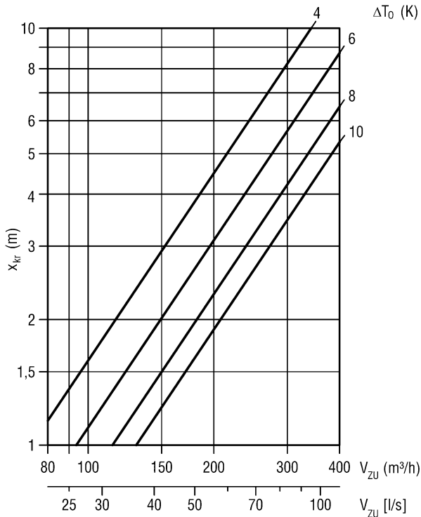
LWD-Q-Z-6-...-00625-125-...
