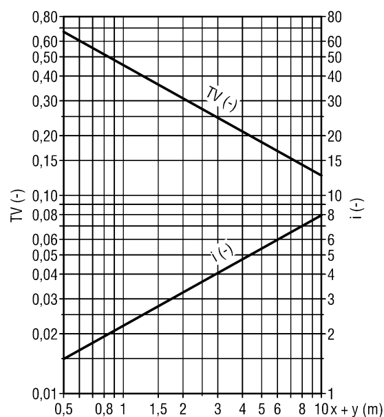
LWD-Q-Z-6-...-01025-225-...
