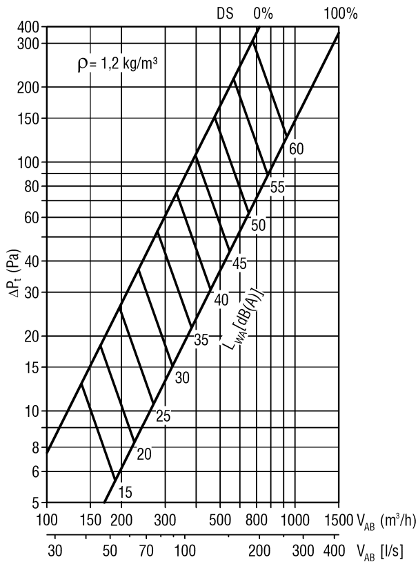
LWD-Q-A-6-...-00625-125-...-AK-80-...-S1
