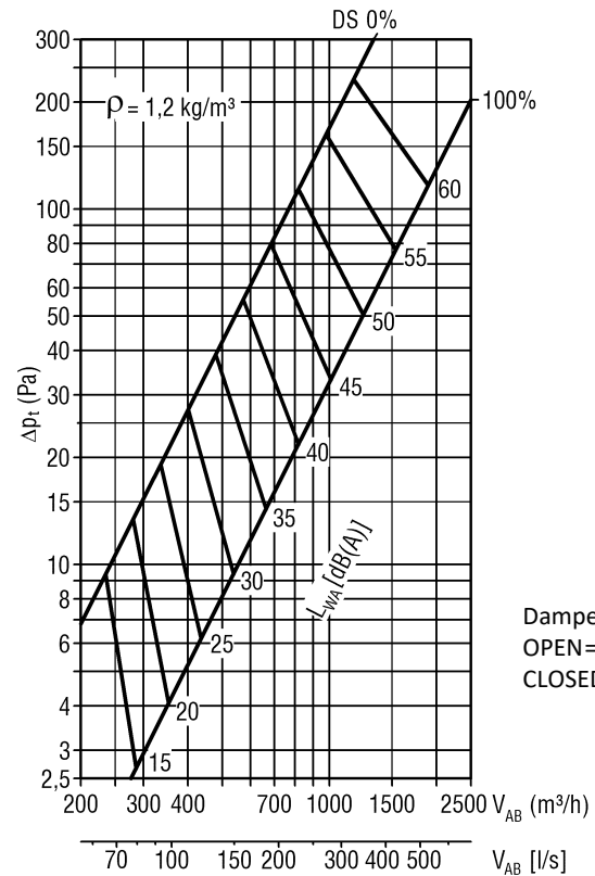
LWD-Q-A-6-...-00625-225-...-AK-80-...-S0
