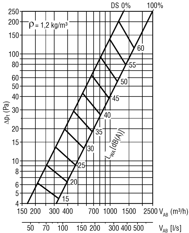
LWD-Q-A-6-...-01025-125-...-AK-80-...-S1
