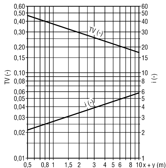
LWD-Q-Z-6-...-001025-125-...
