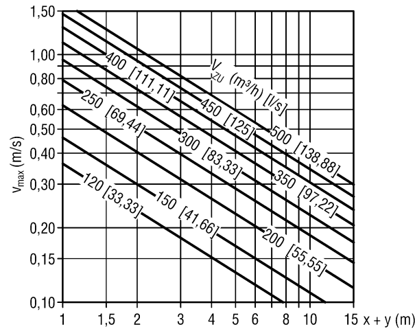
LWD-Q-Z-6-...-01025-225-...
