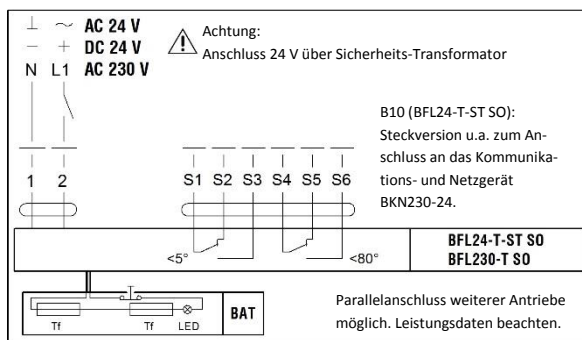
Abbildung 30: Anschluss-Schema B10/B11
