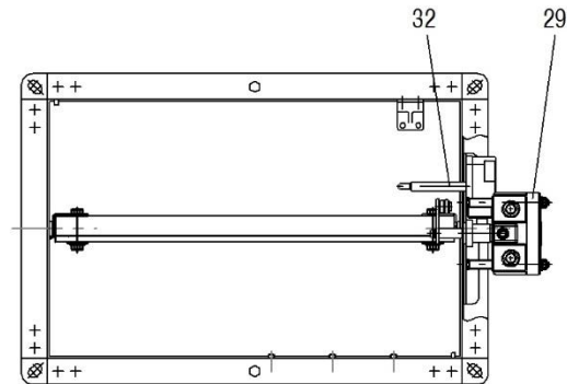
Abbildung 46: Vorderansicht BKP-EN (Federrücklaufantrieb)
