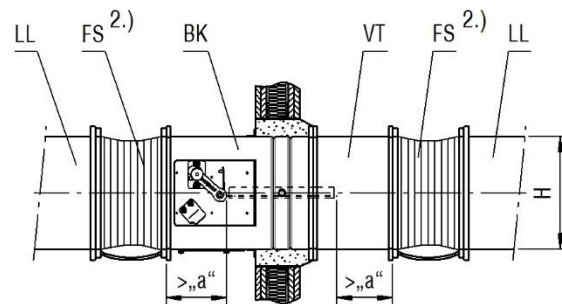
Abbildung 26: Anschlussbeispiel beidseitig mit flexiblem Stützen und Lüftungsleitungen
