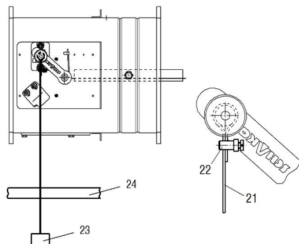
Abbildung 41: Stellungsanzeiger Typ MSZ
