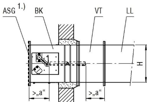
Abbildung 24: Anschlussbeispiel einer einseitig angeordneten Lüftungsleitung und Abschluss-Schutzgitter
