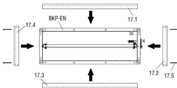
Abbildung 40: BKP-EN mit Einbaurahmen Typ ER-P1 (lose)
