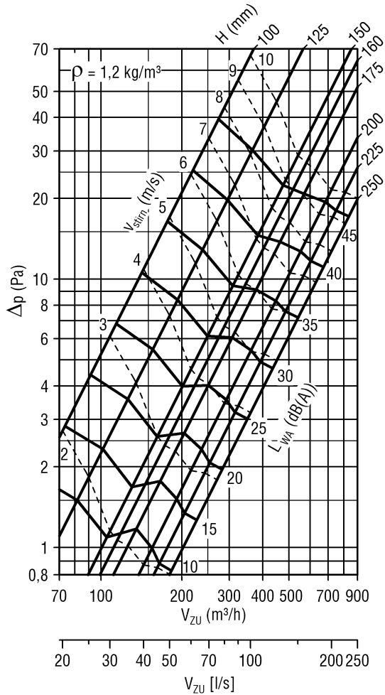
Diagramm 1: Klappenbreite B = 100 mm; Druckverlust und Lautstärke ohne Abschluss-Schutzgitter
