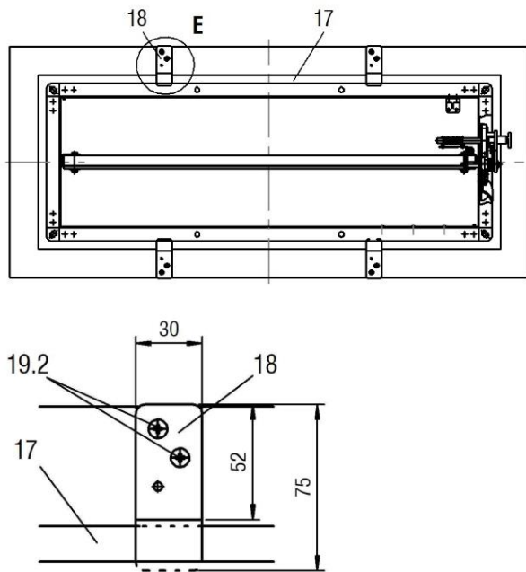
Abbildung 23: Detail Haltetaschen
