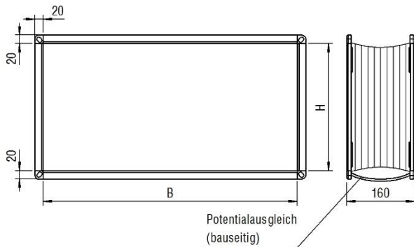
Abbildung 36: Flexibler Stutzen Typ FS
