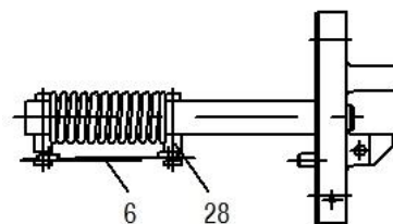
Abbildung 44: Auslöseeinrichtung BKP-EN (Schmelzlot)
