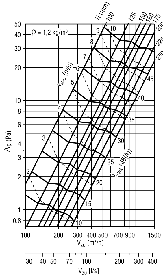
Diagramm 2: Klappenbreite B = 150 mm; Druckverlust und Lautstärke ohne Abschluss-Schutzgitter
