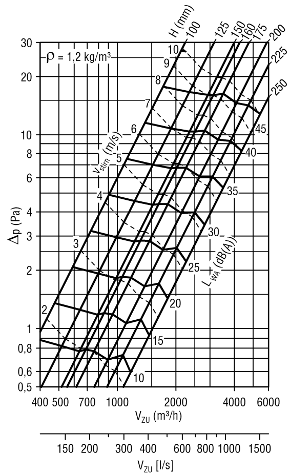
Diagramm 8: Klappenbreite B = 600 mm; Druckverlust und Lautstärke ohne Abschluss-Schutzgitter
