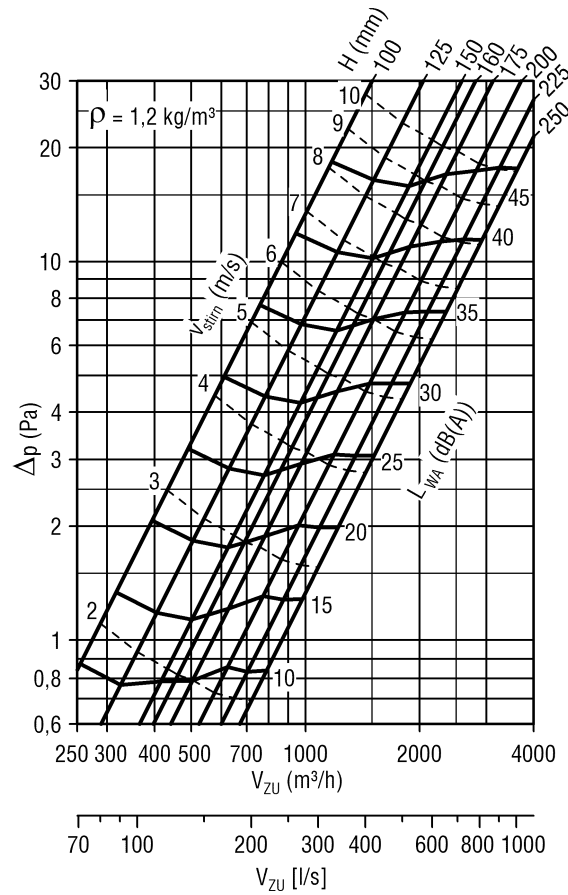
Diagramm 6: Klappenbreite B = 400 mm; Druckverlust und Lautstärke ohne Abschluss-Schutzgitter
