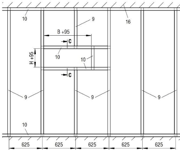
Abbildung 16: Metallständerwerk mit erforderlichen Auswechslungen für BKP-EN mit Einbaurahmen Typ ER-P1
