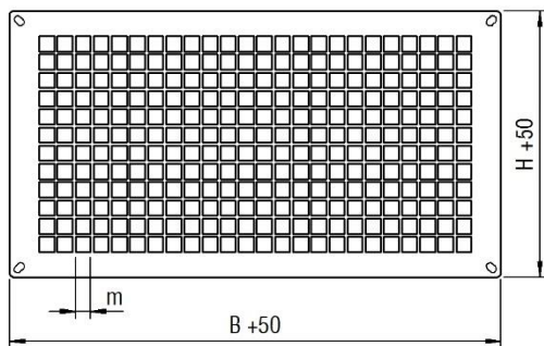
Abbildung 39: Abschluss-Schutzgitter Typ ASG
