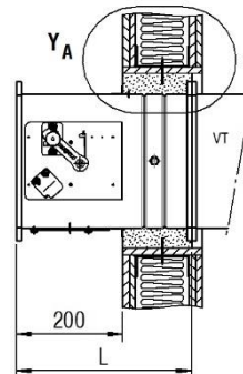
Schnitt A-A
