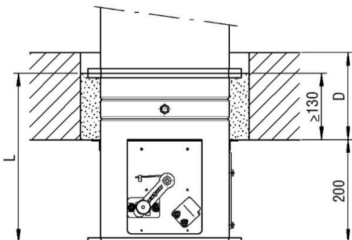
Abbildung 8: Einbaulagen in massiven Decken
