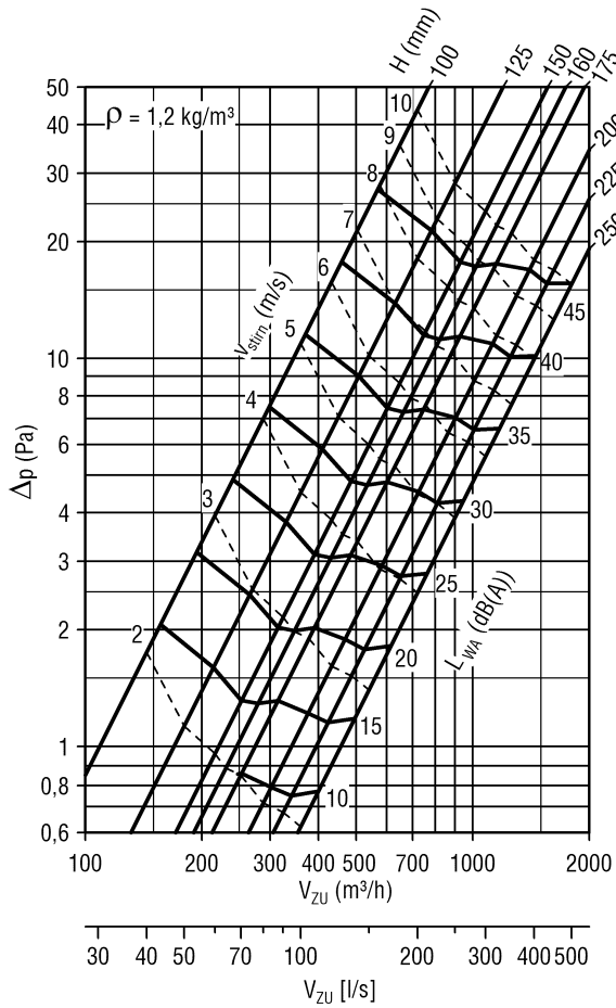
Diagramm 3: Klappenbreite B = 200 mm; Druckverlust und Lautstärke ohne Abschluss-Schutzgitter
