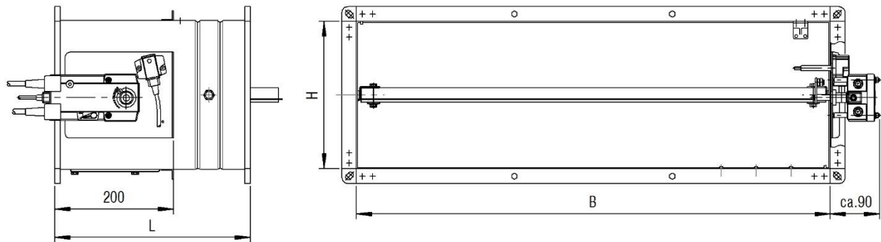
Abbildung 29: BKP-EN mit Federrücklaufantrieb B10/B11
