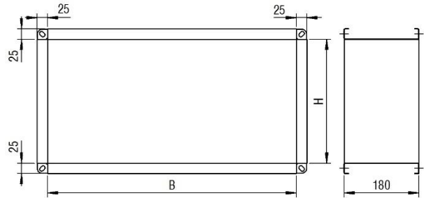
Abbildung 37: Verlängerungsteil Typ VT
