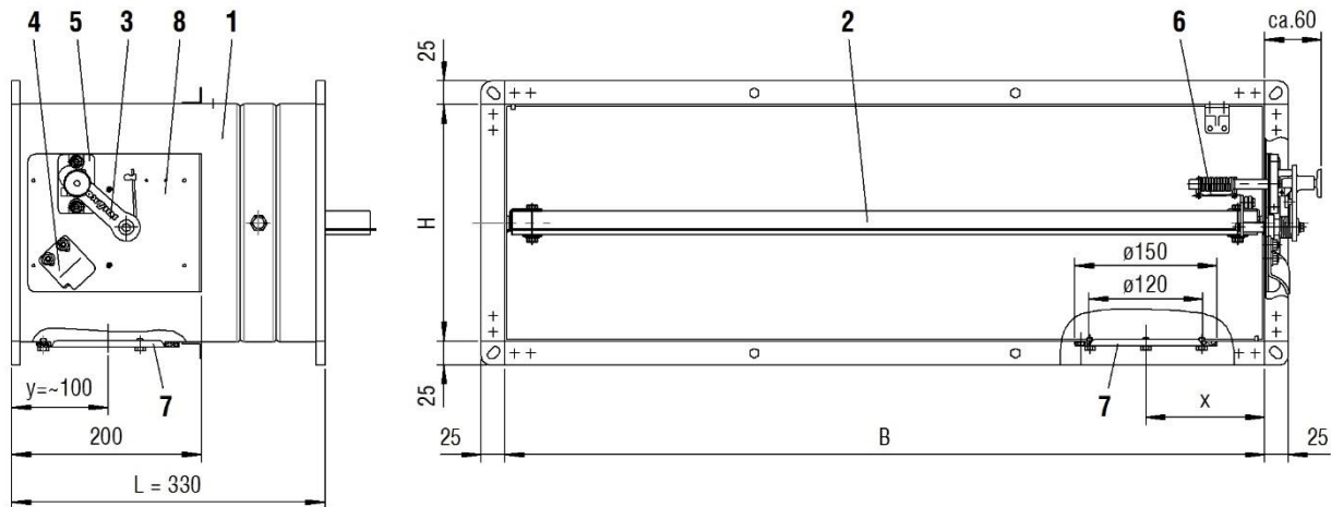
Abbildung 1: Abmessungen BKP-EN
