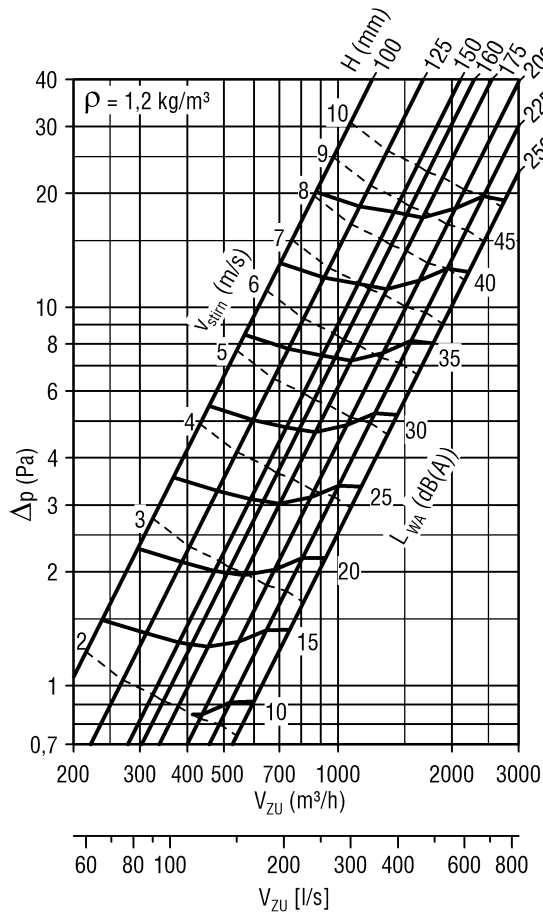
Diagramm 5: Klappenbreite B = 300 mm; Druckverlust und Lautstärke ohne Abschluss-Schutzgitter
