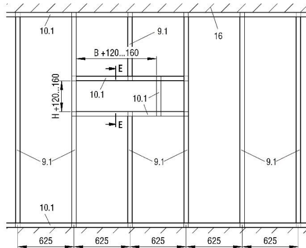
Abbildung 19: Metallständerwerk mit erforderlichen Auswechslungen für Nasseinbau (Schachtwand)
