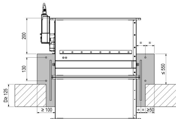
Abbildung 12: Einbau in massive Decken mit Betonsockel, Schnitt
