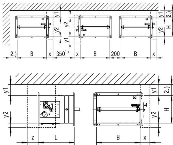
Abbildung 5: Mindestabstände zu Wänden und Decken sowie BKP-EN zueinander
