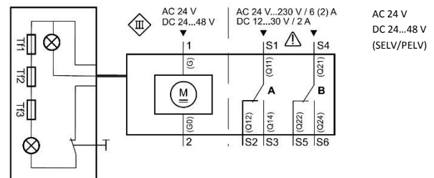
Abbildung 33: Anschluss-Schema S00
