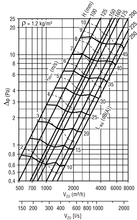
Klappenbreite B = 800 mm
