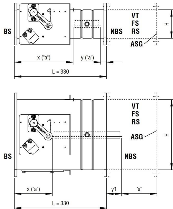
Abbildung 4: Klappenblattüberstände
