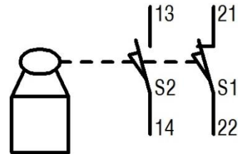
Abbildung 27: Schaltbild Endschalter Typ ES
