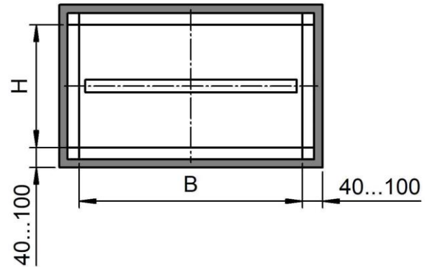
Abbildung 7: Ringspaltmaße vollständige Ausmörtelung in massiven Wänden
