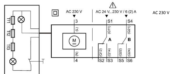
Abbildung 34: Anschluss-Schema S01
