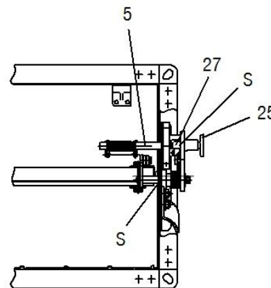
Abbildung 43: Vorderansicht BKP-EN (Handauslösung)
