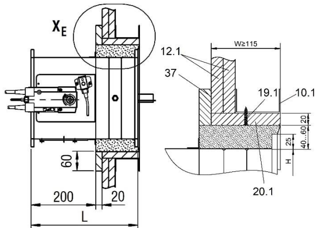
Abbildung 20: Wandbeplankung und Aufdoppelung (Schachtwand)
