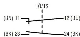
Abbildung 28: Schaltbild Endschalter Typ ES-Ex
