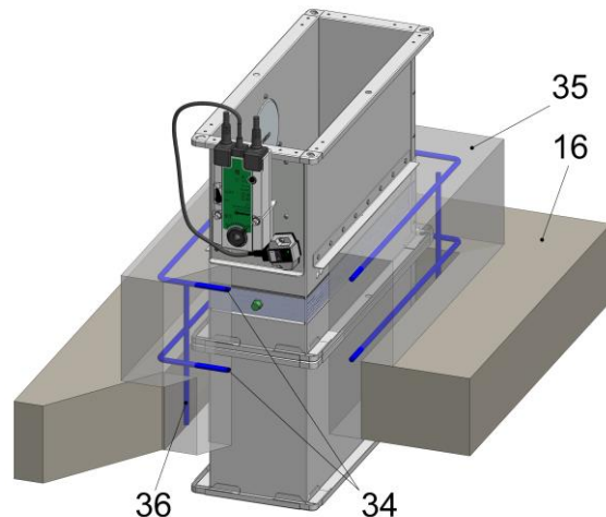
Abbildung 11: Einbau in massive Decken mit Betonsockel
