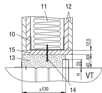
Abbildung 14: Nasseinbau in leichte Trennwand (F90)
