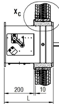
Abbildung 16: Metallständerwerk mit erforderlichen Auswechslungen für BKP-EN mit Einbaurahmen Typ ER-P1
