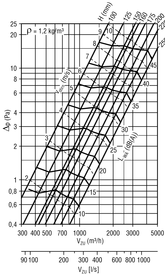
Klappenbreite B = 500 mm
