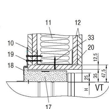
Abbildung 18: Trockeneinbau mit Einbaurahmen Typ ER-P1 (Schnitt) in leichte Trennwand (F90)
