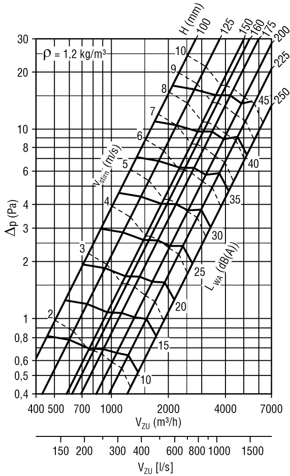
Klappenbreite B = 700 mm
