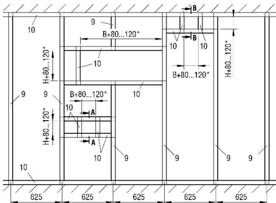
Abbildung 14: Nasseinbau in leichte Trennwand (F90)
