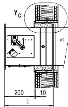
Abbildung 18: Trockeneinbau mit Einbaurahmen Typ ER-P1 (Schnitt) in leichte Trennwand (F90)
