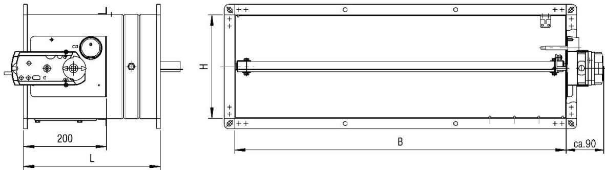
Abbildung 31: BKP-EN mit Federrücklaufantrieb S00/S01
