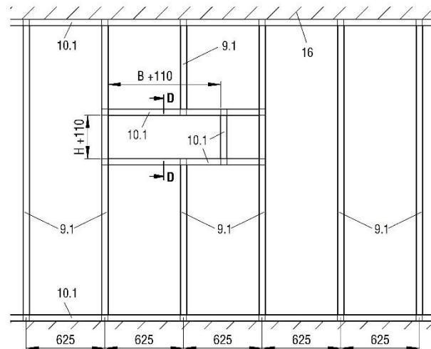
Abbildung 21: Metallständerwerk mit erforderlichen Auswechslungen für Trockeneinbau mit Einbaurahmen ER-P1
