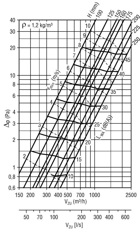
Diagramm 4: Klappenbreite B = 250 mm; Druckverlust und Lautstärke ohne Abschluss-Schutzgitter
