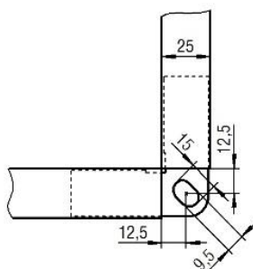
Abbildung 3: Einzelheit A - Eckwinkel
