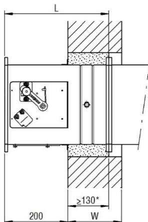
Abbildung 6: Einbaulagen in massiven Wänden
