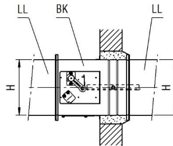
Abbildung 25: Anschlussbeispiel beidseitig mit Lüftungsleitungen
