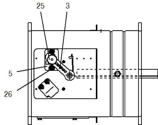
Abbildung 42: Seitenansicht BKP-EN (Handauslösung)
