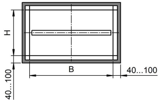
Abbildung 9: Ringspaltmaße vollständige Ausmörtelung in massiven Decken
