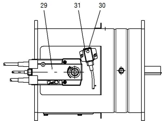
Abbildung 45: Seitenansicht BKP-EN (Federrücklaufantrieb)
